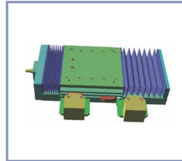
Tavola TV1 Supporto elettromandrino di macchina speciale per taglio profilati alluminio. Corsa 150 mm
